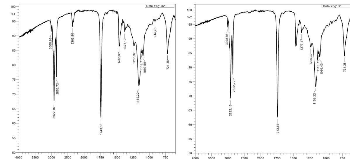
2-chizma. Dog'langan va dog'lanmagan kungaboqar yog'ida yorug'lik yutilish koeffitsiyentining to'lqin uzunligiga bog'liqligi.
