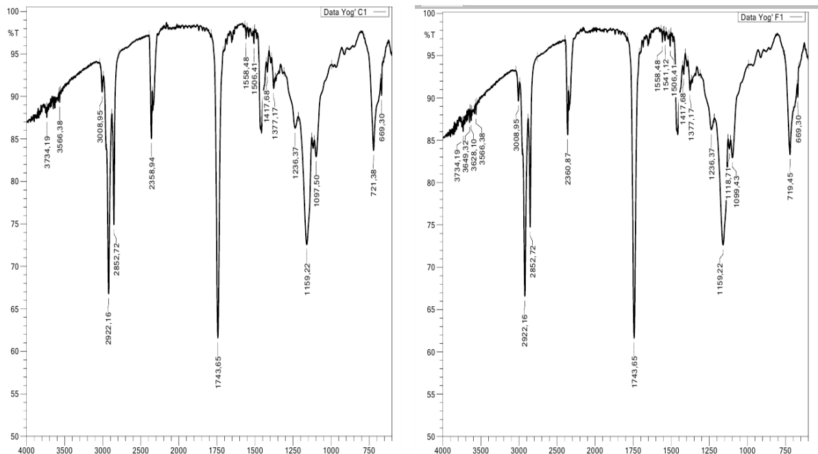
1-chizma. Dog'langan va dog'lanmagan paxta yog'ida yorug'lik yutilish koeffitsiyentining to'lqin uzunligiga bog'liqligi.
