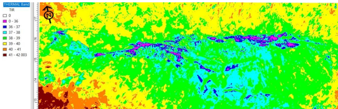
2-rasm. Issiqlik infraqizil diapazonida olingan kosmik suratni yer yuzasi issiqlik harorat xaritasi (Kuljuktog' hududi)
