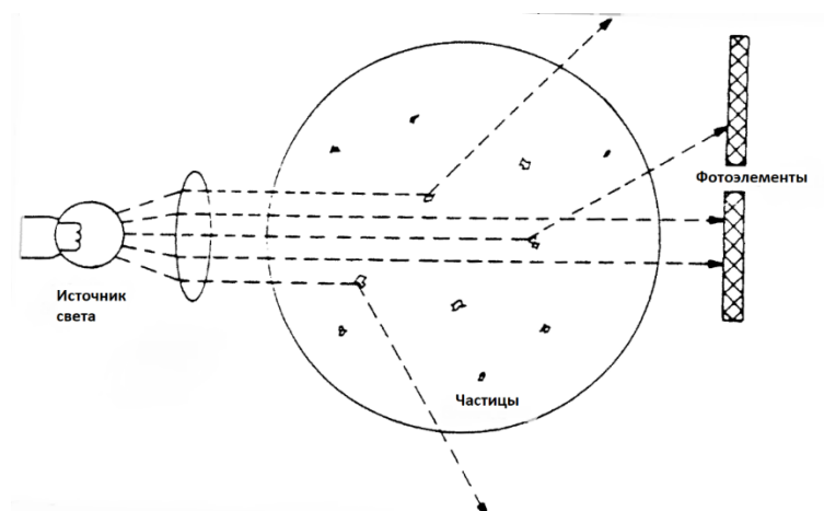
Рисунок 1. Принцип оптического измерения концентрации активного ила.
