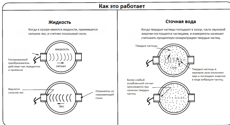
Рисунок 2 - Общая схема ультразвукового анализатора концентрации твердых веществ.
